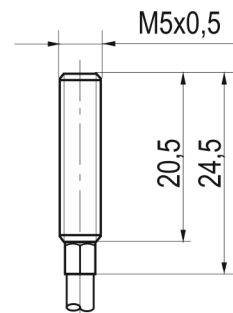
Габаритный чертеж
